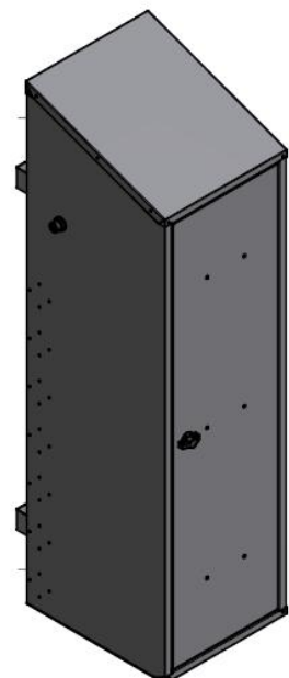
Für 7 Paar Handschuhe (Wandbefestigung) Maße BxTxH 350 x 400 x 1110/1220 mm
