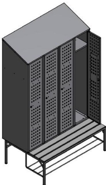
Beispiel F-034 ES4/MS mit zusätzlicher Schuhablage unter der Sitzbank
